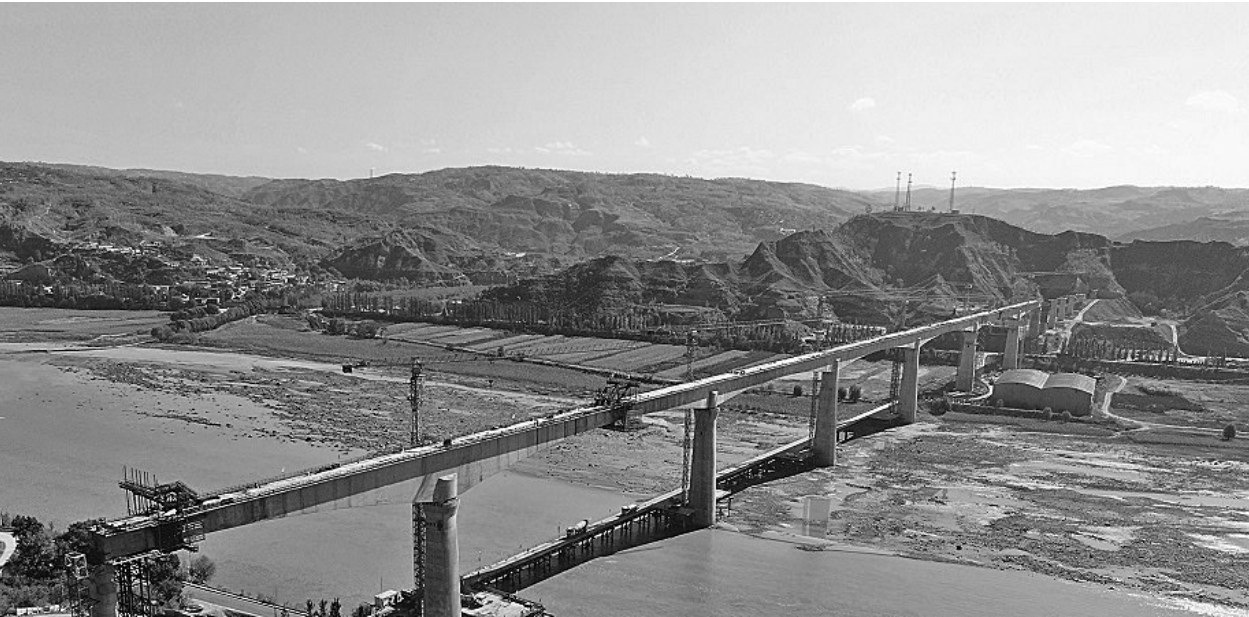
10月10日，由陕西铁路物流集团冯弘铁路公司建设、铁一院勘察设计、中铁十八局承建的神瓦铁路黄河特大桥合龙。作为神瓦铁路全线唯一一座跨越黄河的桥梁，其合龙标志着陕晋能源大通道的重难点控制性工程取得关键突破。
